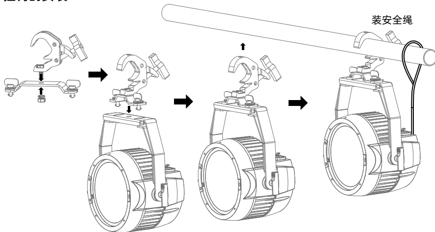
挂钩的安装
