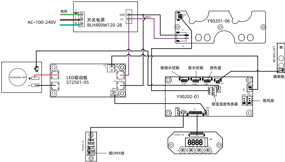
九、控制线路图
