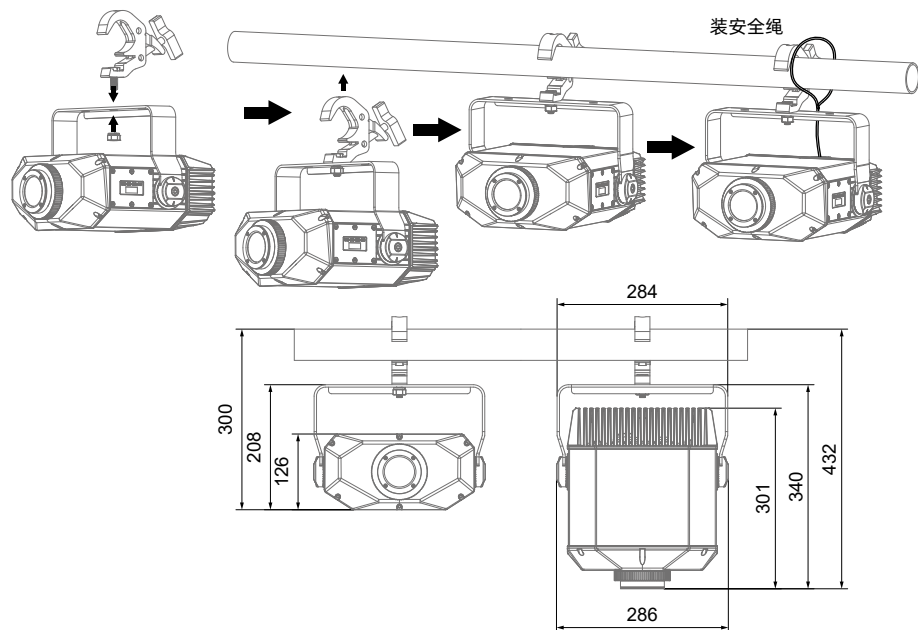
挂钩的安装
